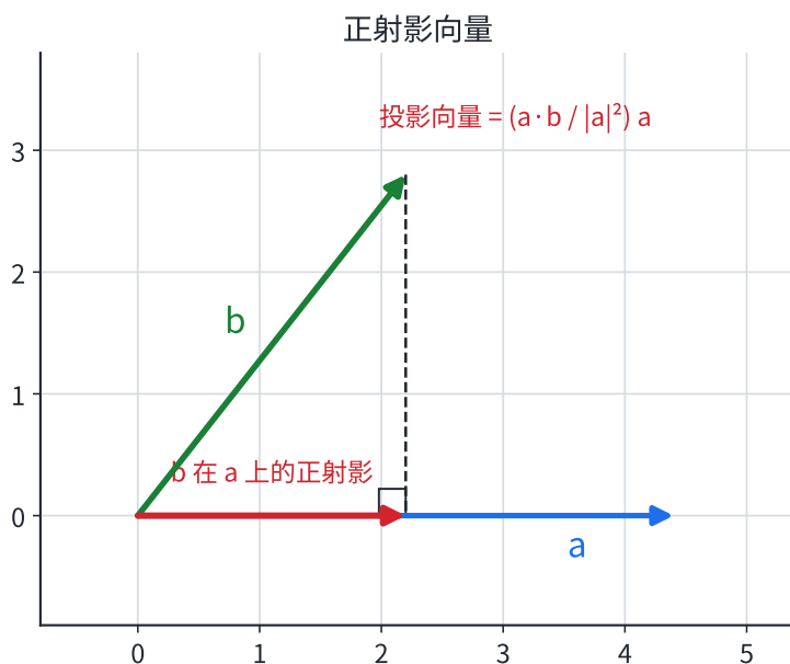
圖 3-5： \vec{b} 在 \vec{a} 上的正射影。從 \vec{b} 的尖端對 \vec{a} 所在直線作垂線，落點與原點之間沿 \vec{a} 方向的那支紅色向量，即正射影向量 \left( \frac{\vec{a} \cdot \vec{b}}{|\vec{a}|^2} \right) \vec{a} 。
