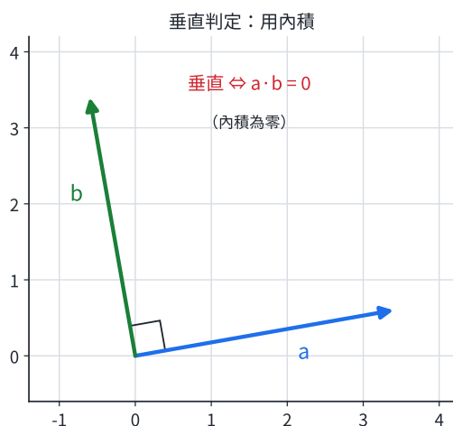
圖 3-4：兩種判定剛好相反。左——垂直用內積： \vec{a} \perp \vec{b} \iff \vec{a} \cdot \vec{b} = 0 （圖中直角記號）；右——平行用行列式： \vec{a} \parallel \vec{b} \iff a_1 b_2 - a_2 b_1 = 0 （兩向量落在同一條直線上，同向或反向）。
