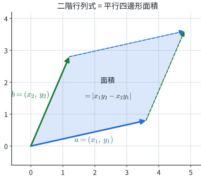
圖 3-6：以 \vec{a} = (x_1, y_1) 、 \vec{b} = (x_2, y_2) 為鄰邊的平行四邊形，其面積等於二階行列式的絕對值 |x_1y_2 - x_2y_1| 。
