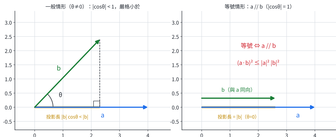
圖 3-7：柯西不等式的幾何意義。左——當 \vec{a} 、 \vec{b} 夾角 \theta \neq 0 時， \vec{b} 在 \vec{a} 上的投影長 |\vec{b}| \cos \theta 嚴格小於 |\vec{b}| （因 |\cos \theta| < 1 ），故 (\vec{a} \cdot \vec{b})^2 < |\vec{a}|^2 |\vec{b}|^2 ；右——當 \vec{a} \parallel \vec{b} ( \theta = 0 ) 時投影長等於 |\vec{b}| ，不等式取等號。柯西不等式正是「 |\cos \theta| \leq 1 」的代數化身。
